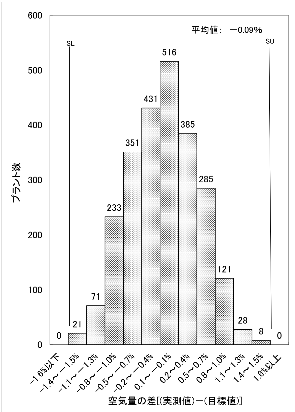
図-8 令和6年度空気量の適合性(実地調査) N=2,450
