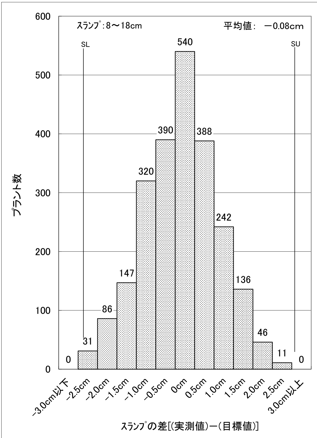
図-7 令和6年度スラップの適合性(実地調査) N=2,337
