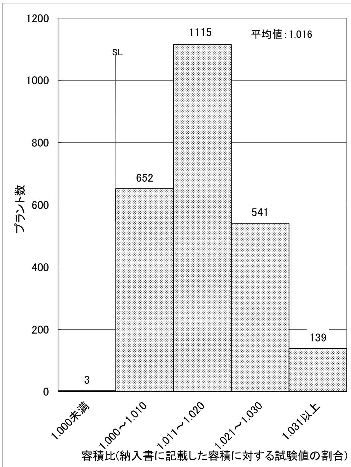
図-9 令和6年度容積の適合性(実地調査) N=2,450
