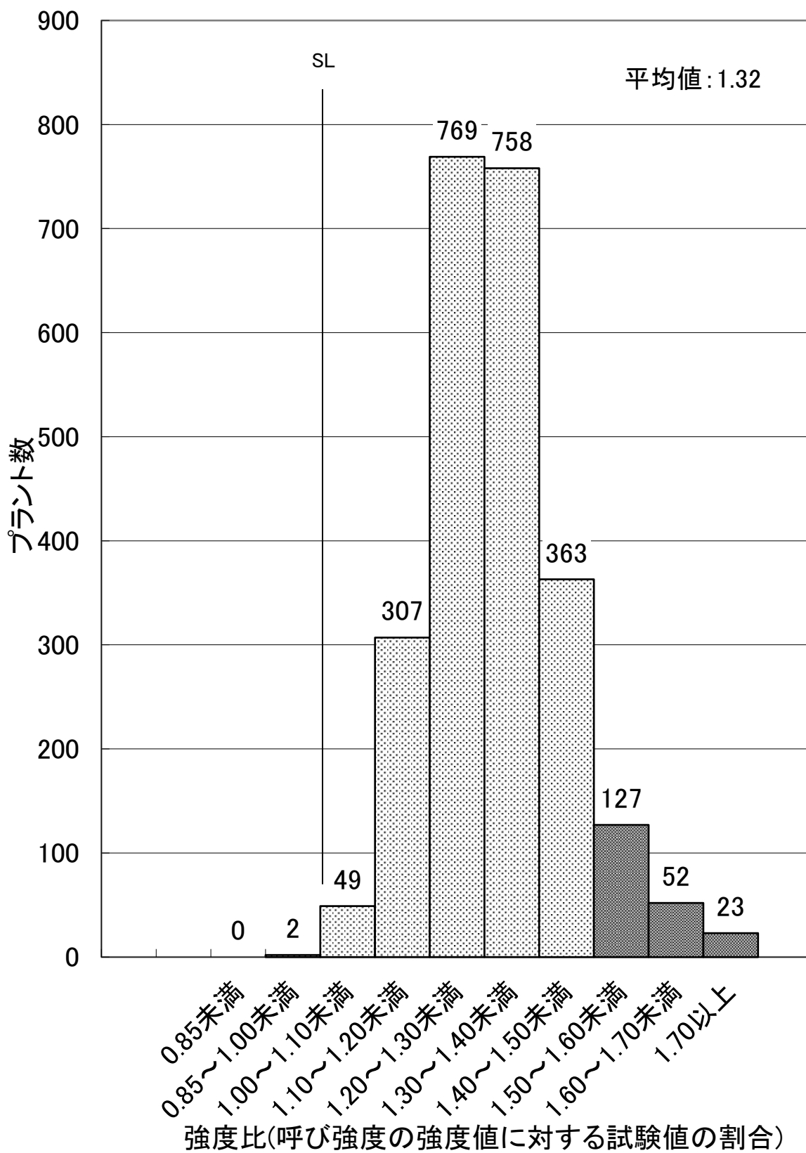
図-6 令和6年度圧縮強度の適合性 N=2,450
