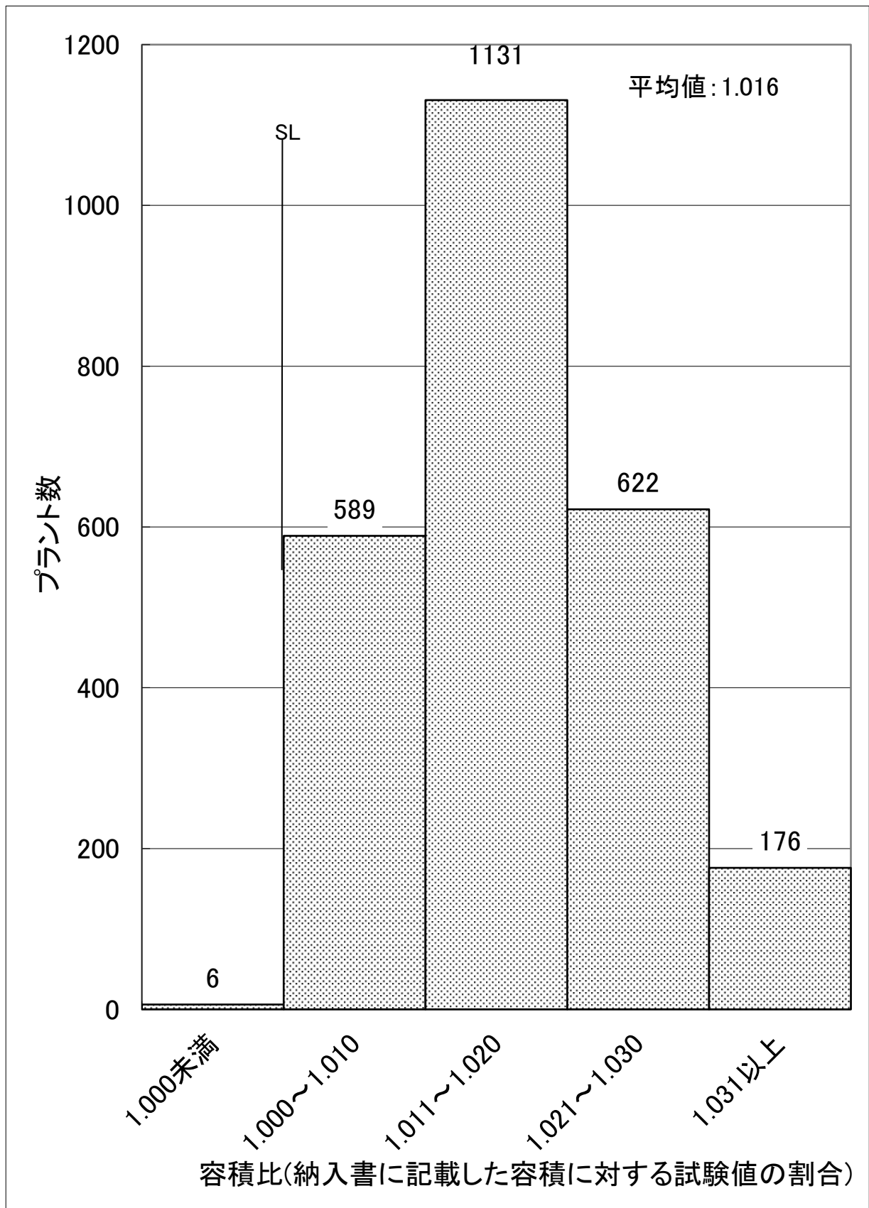
図-9 令和3年度容積の適合性(実地調査) N=2,524
