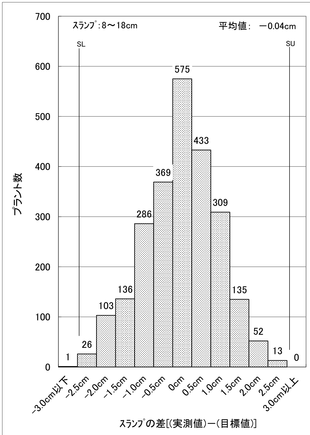
図-7 令和3年度スランプの適合性(実地調査)N=2,438
