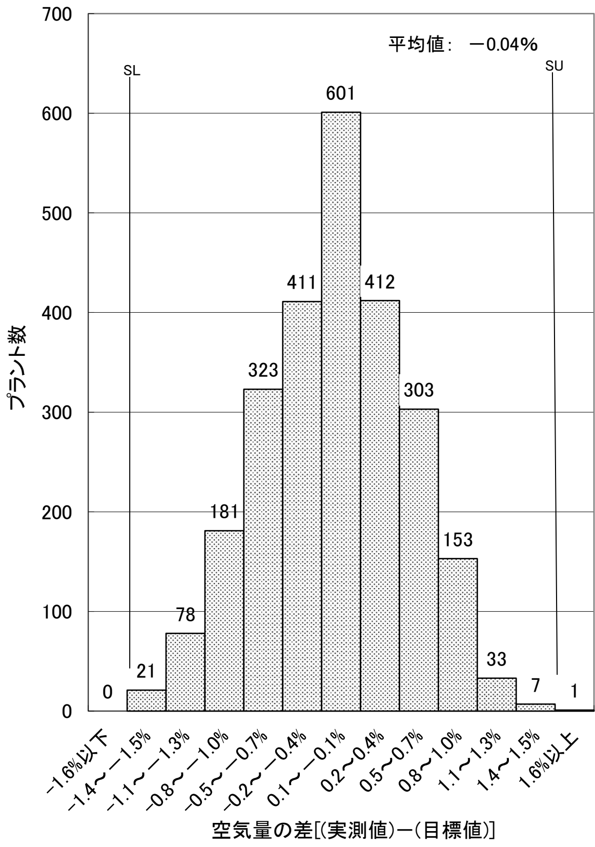
図-8 令和3年度空気量の適合性(実地調査) N=2,524
