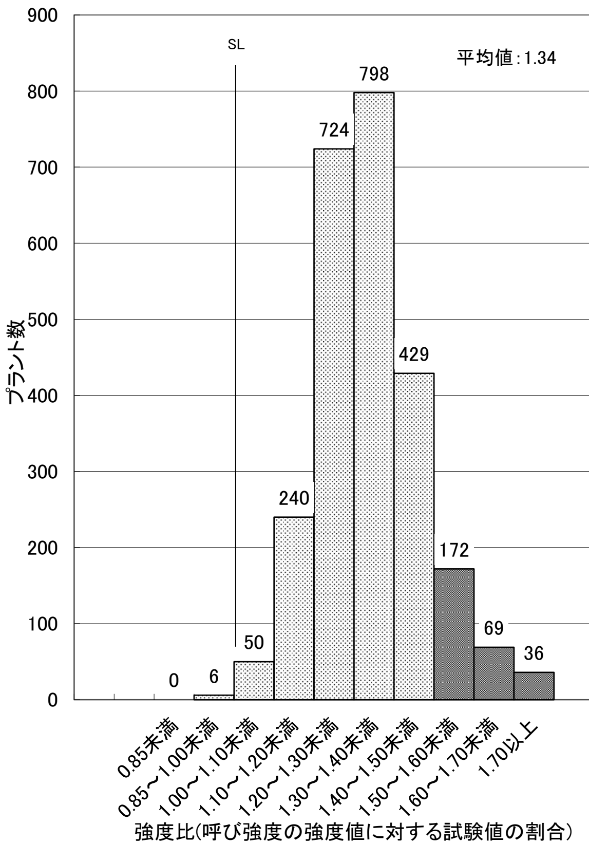
図-6 令和3年度圧縮強度の適合性 N=2,524
