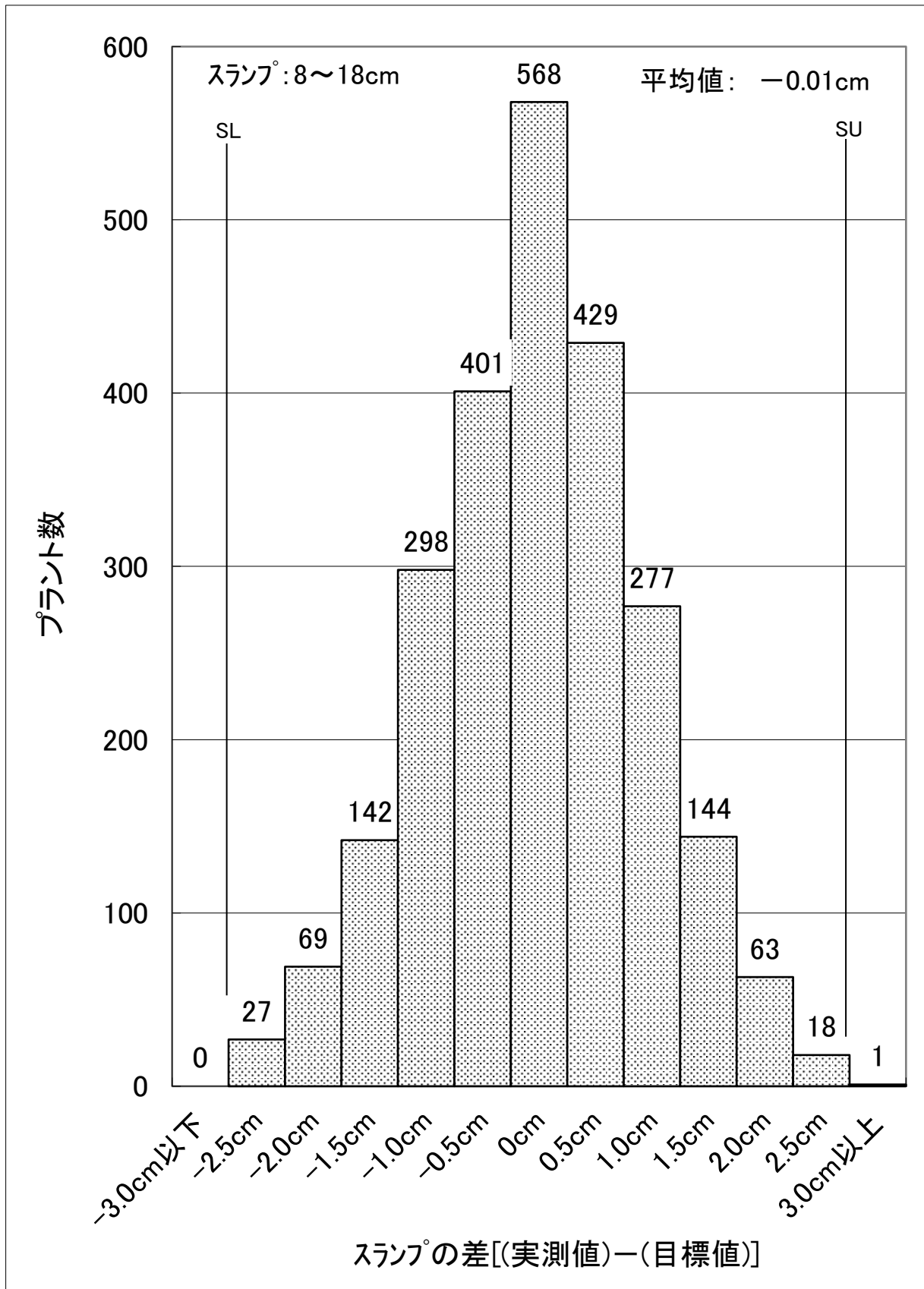
図-7 令和2年度スランプの適合性(実地調査)N=2,437
