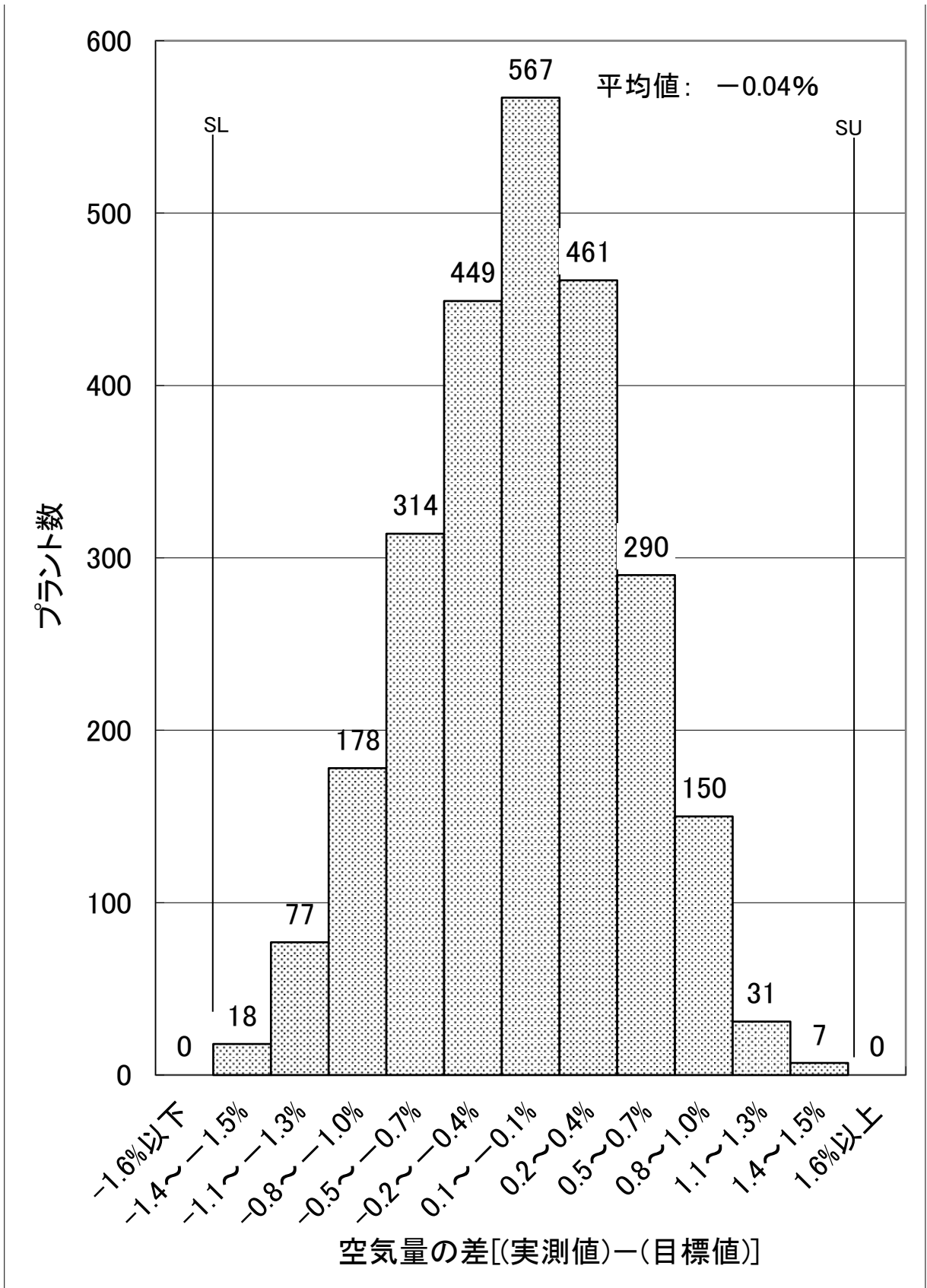
図-8 令和2年度空気量の適合性(実地調査) N=2,542
