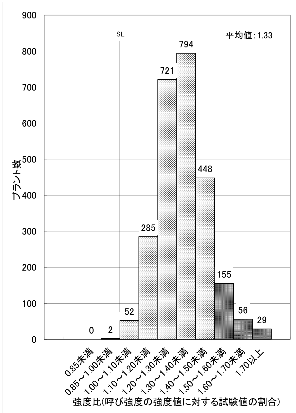
図-6 令和2年度圧縮強度の適合性 N=2,542
