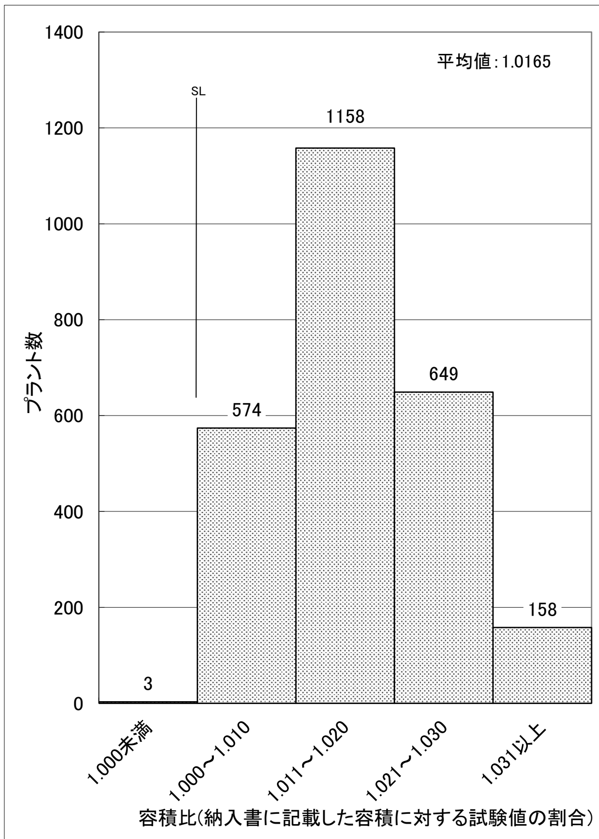
図-9 令和2年度容積の適合性(実地調査) N=2,542
