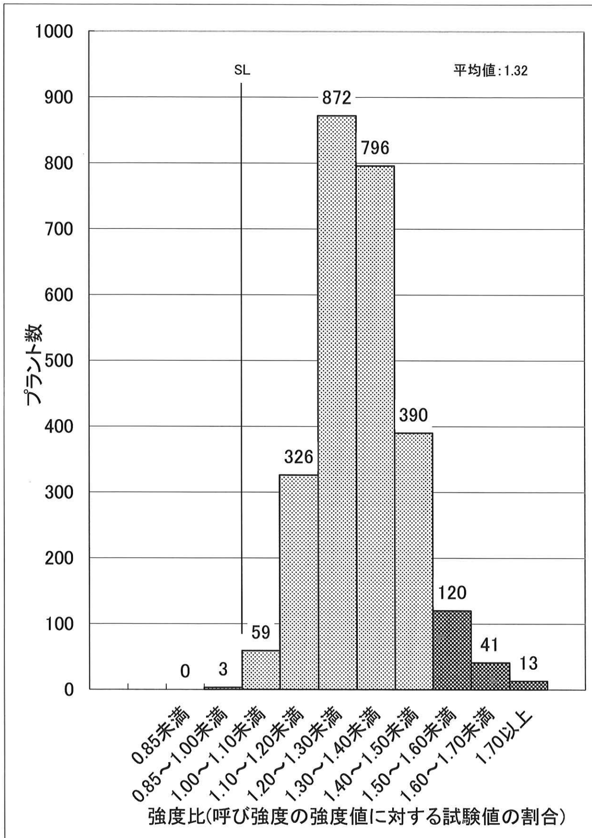
図-6 平成28年度圧縮強度の適合性 N=2,620
