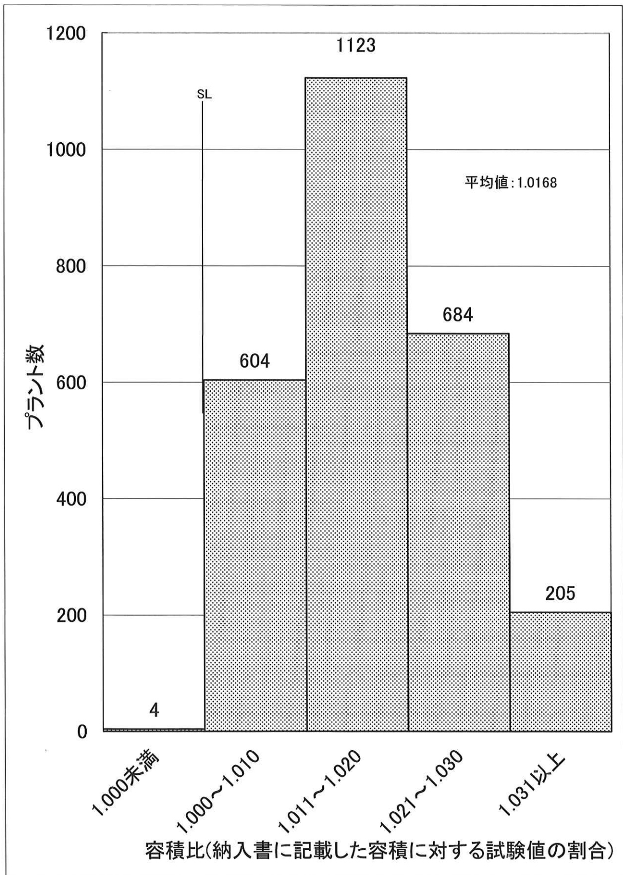
図-9 平成28年度容積の適合性(実地調査) N=2,620
