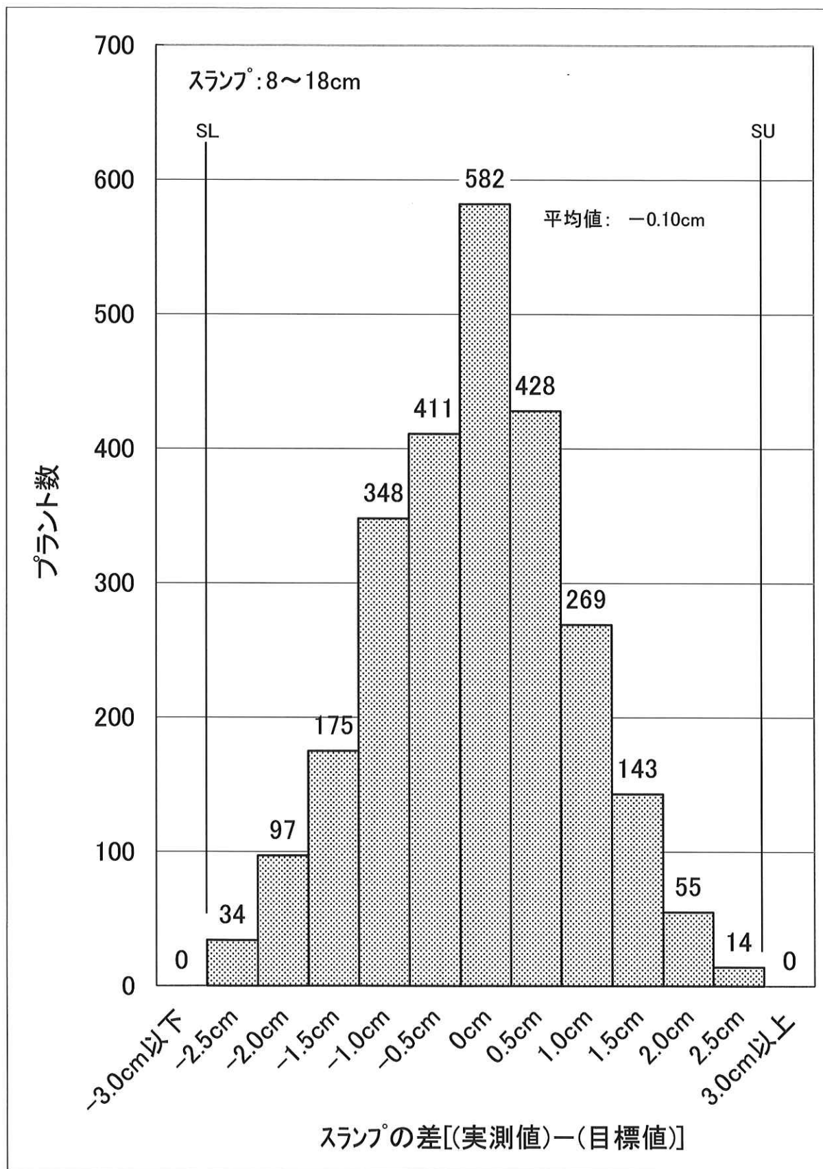
図-7 平成28年度スランプの適合性(実地調査)N=2,556
