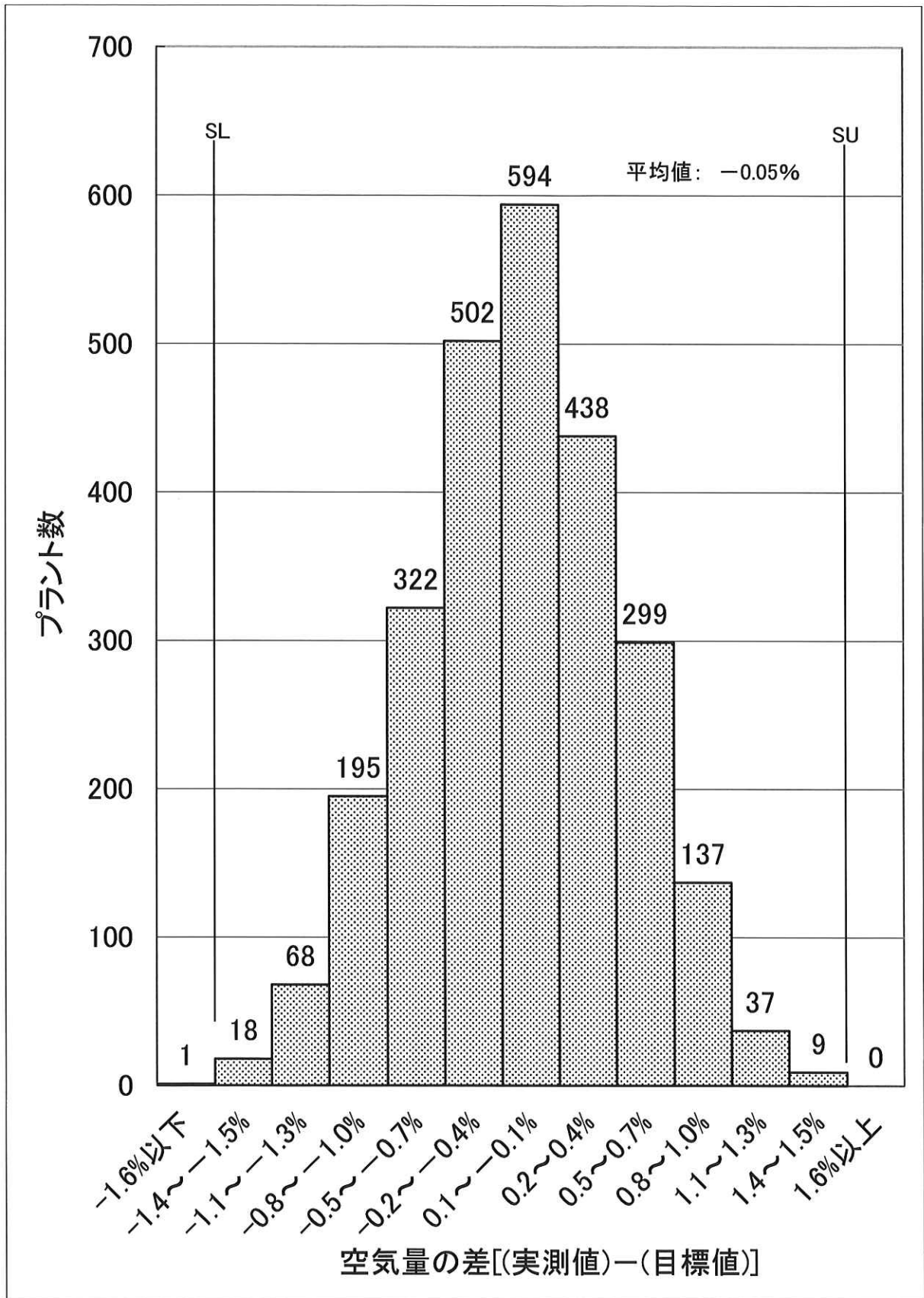
図-8 平成28年度空気量の適合性(実地調査)N=2,620
