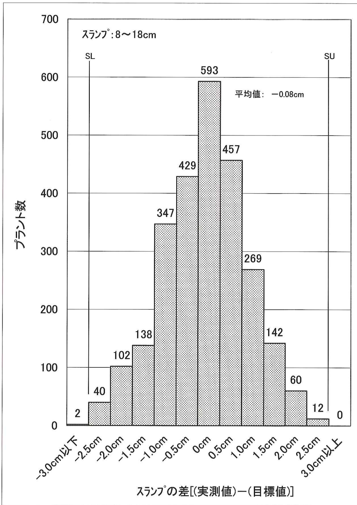
図-7 平成27年度スランプの適合性(実地調査)N=2,591
