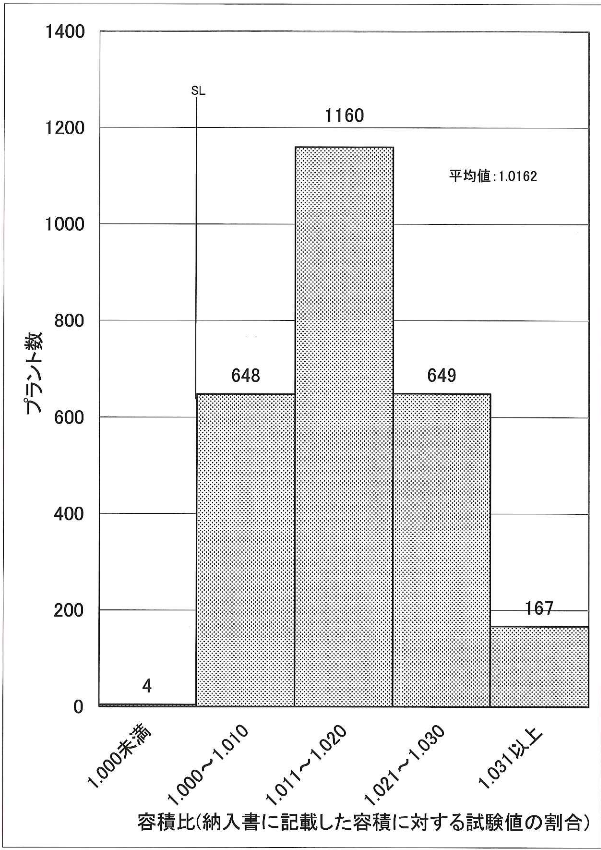
図-9 平成27年度容積の適合性(実地調査)N=2,628
