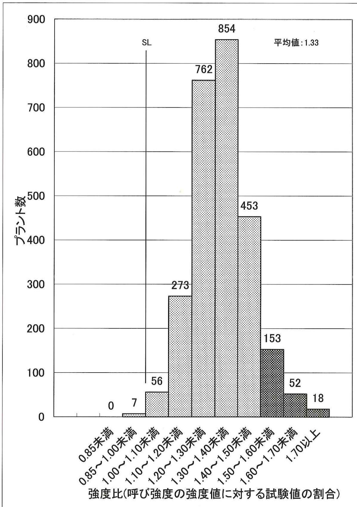
図-6 平成27年度圧縮強度の適合性 N=2,628
