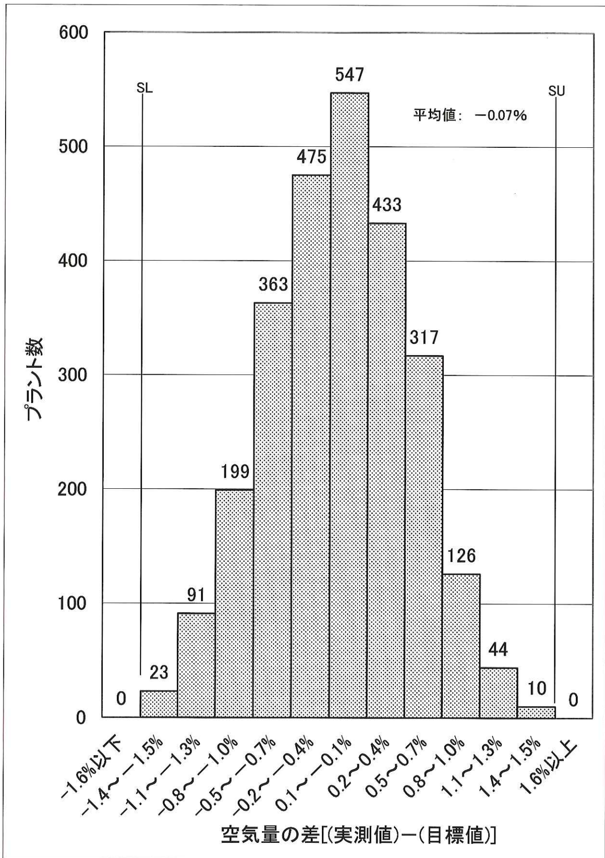
図-8 平成27年度空気量の適合性(実地調査)N=2,628
