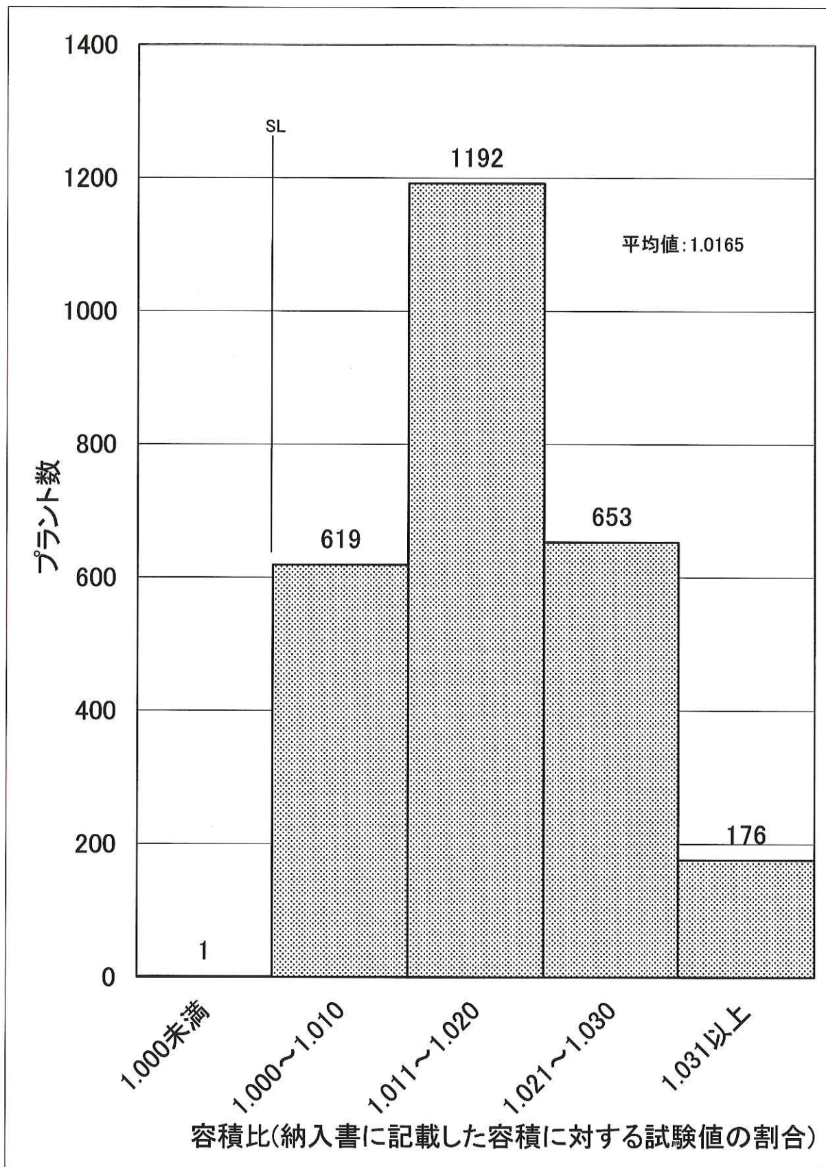
図-9 平成26年度容積の適合性(実地調査)N=2,641
