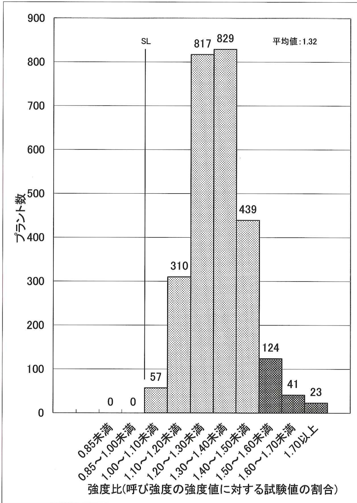
図-6 平成26年度圧縮強度の適合性 N=2,640
