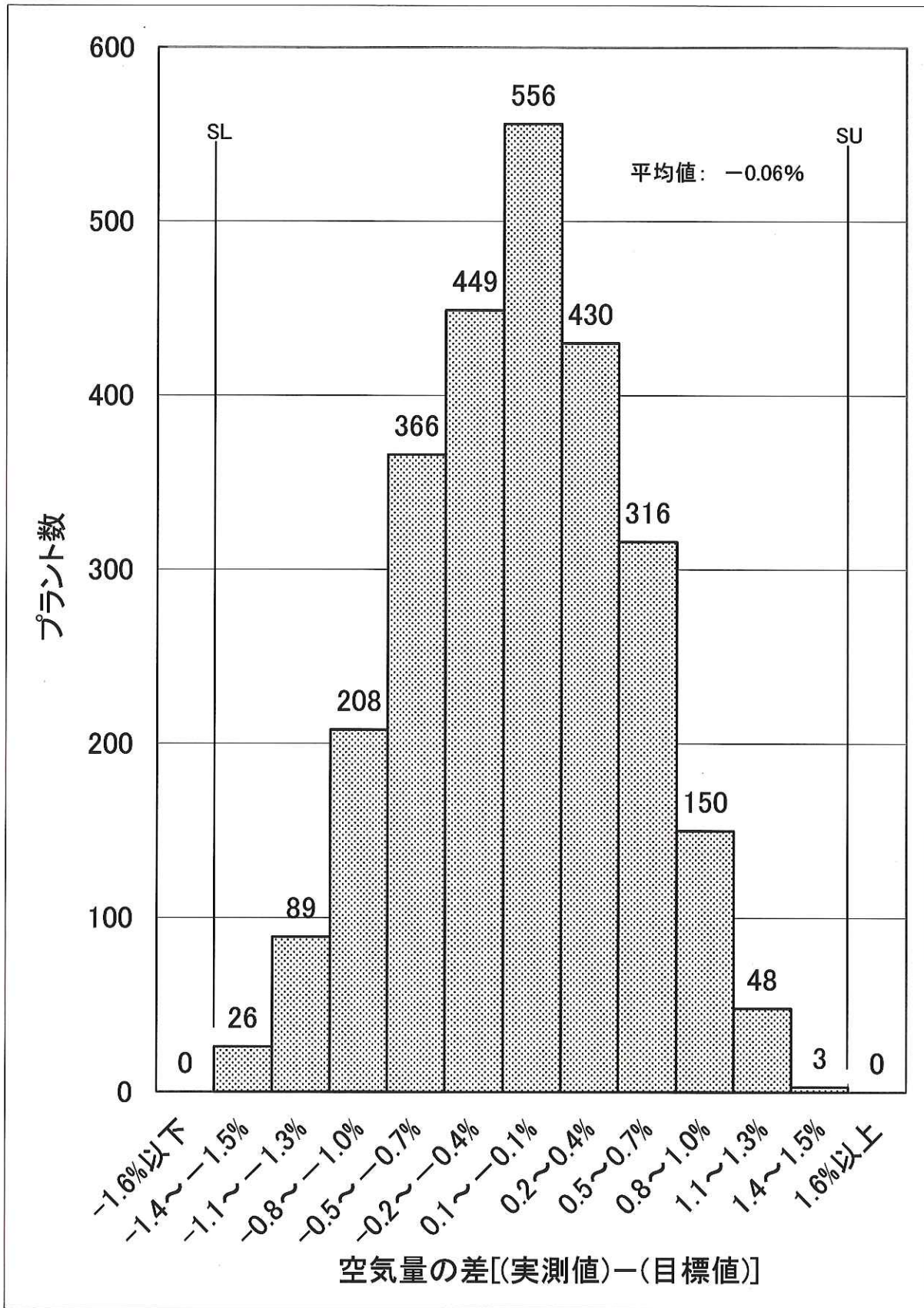
図-8 平成26年度空気量の適合性(実地調査)N=2,641
