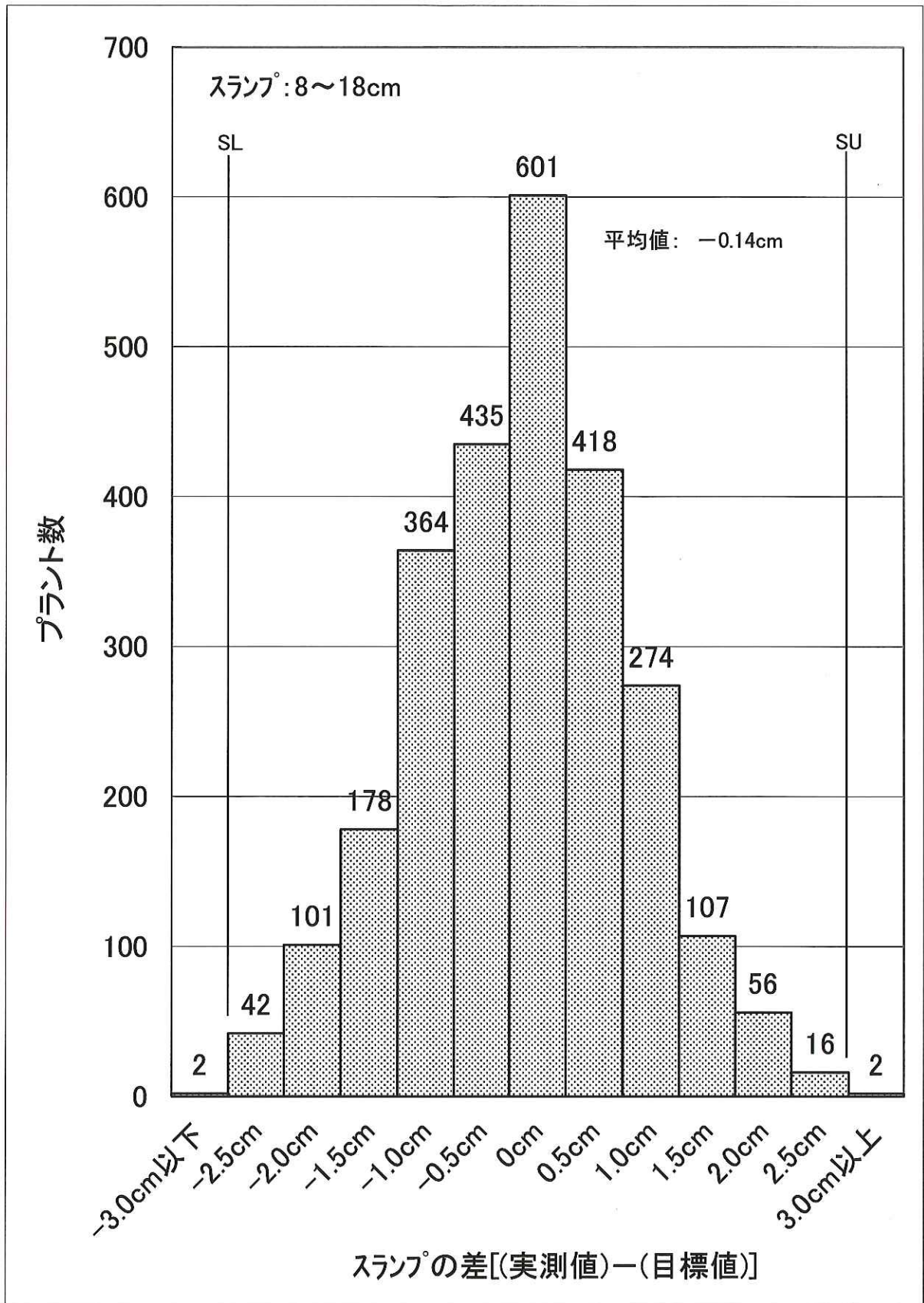
図-7 平成26年度スランプの適合性(実地調査) N=2,596
