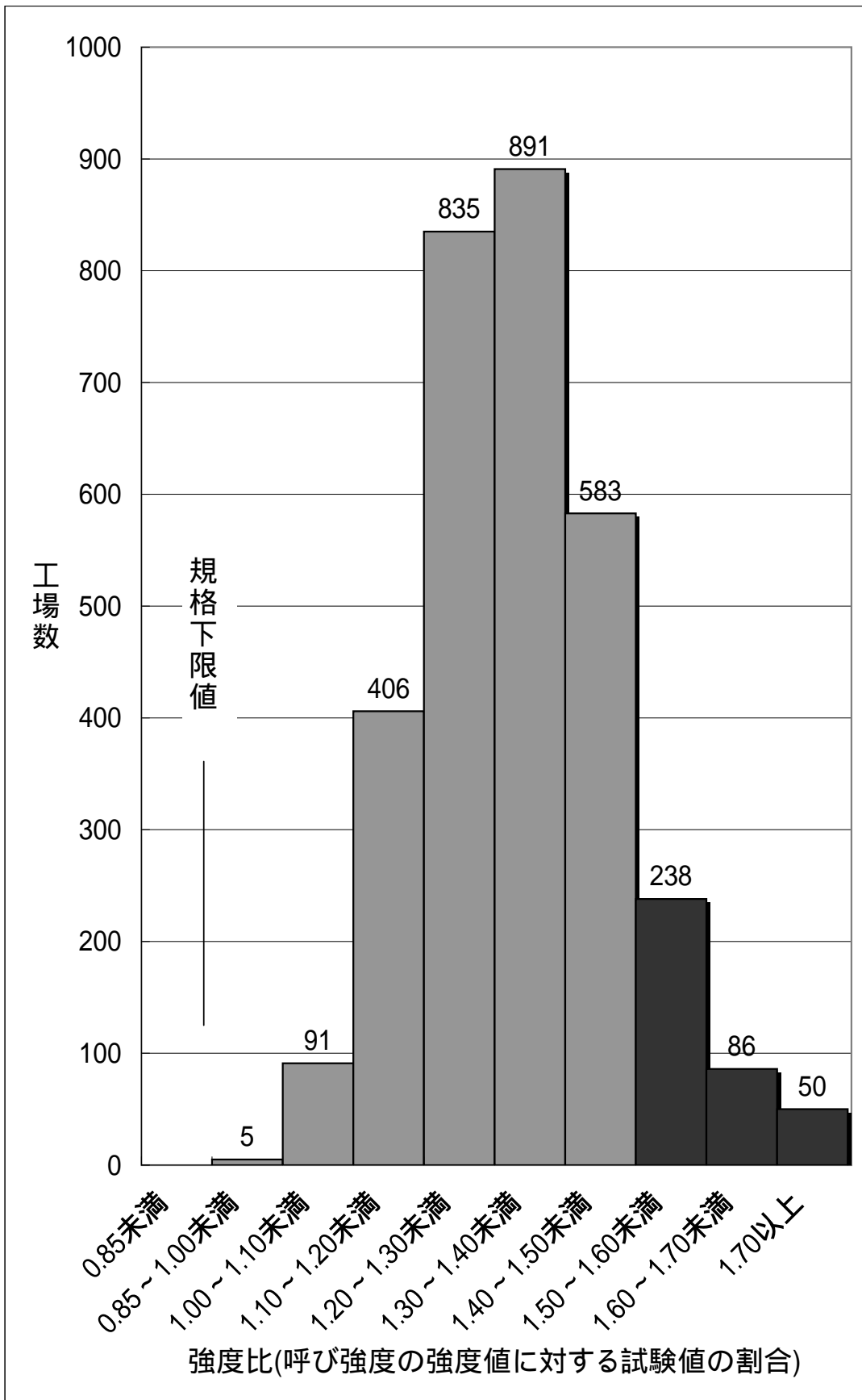
図-5 平成14年度 コンクリート圧縮強度の適合性 ( 実地調査 )
