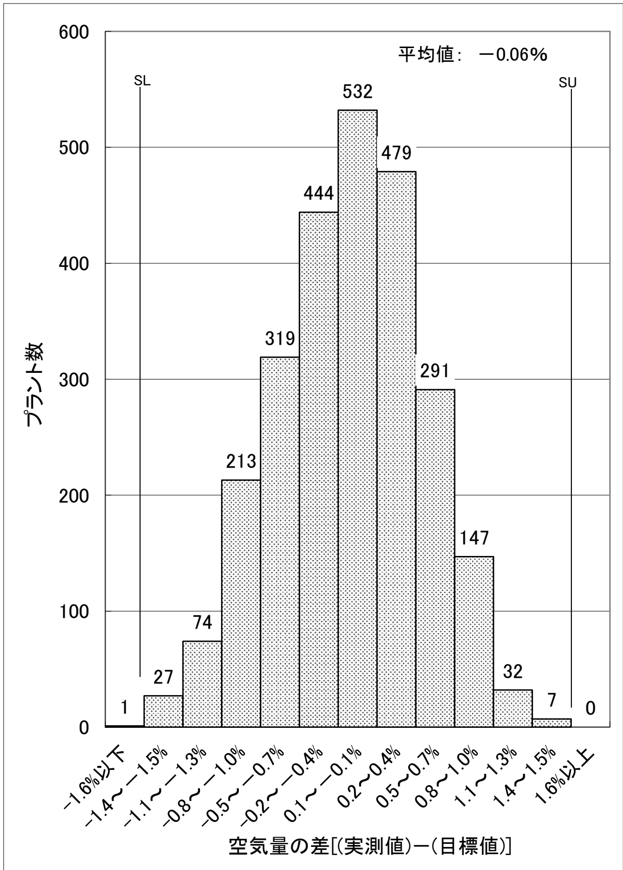
図-8 2019年度空気量の適合性(実地調査) N=2,566
