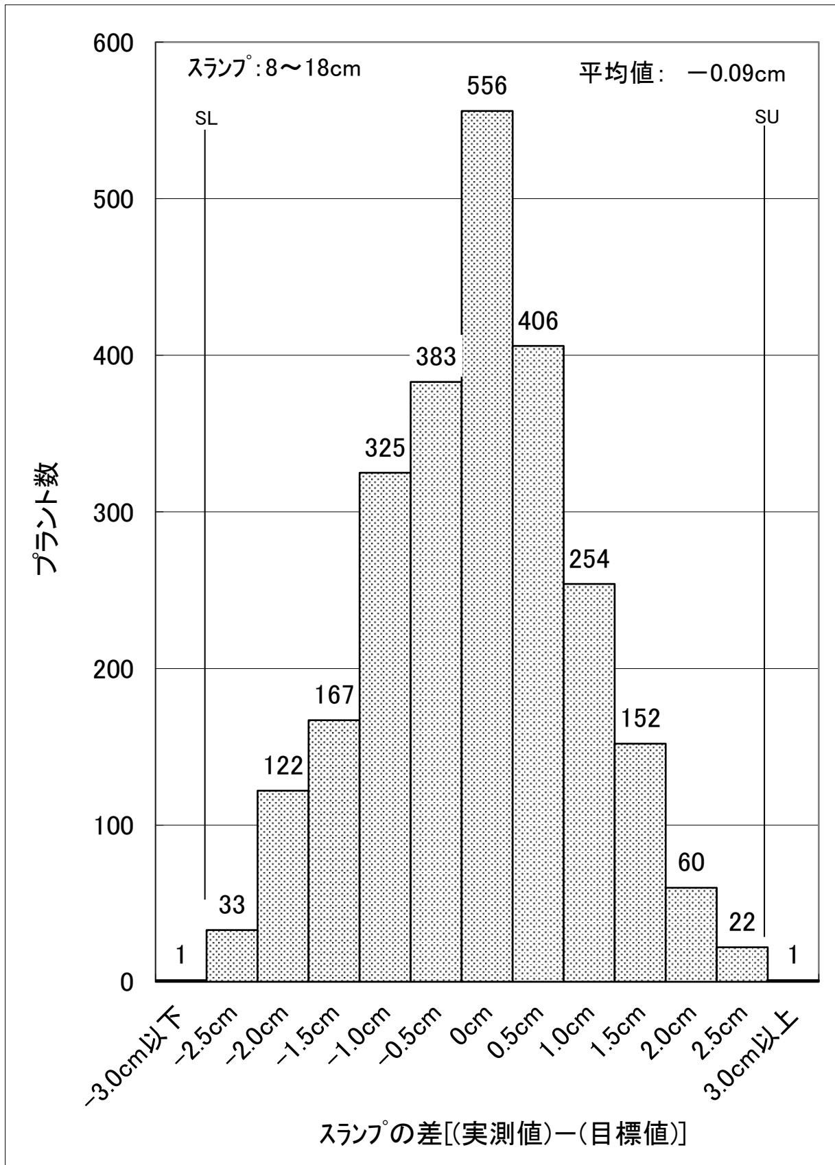
図-7 2019年度スランプの適合性(実地調査)N=2,482
