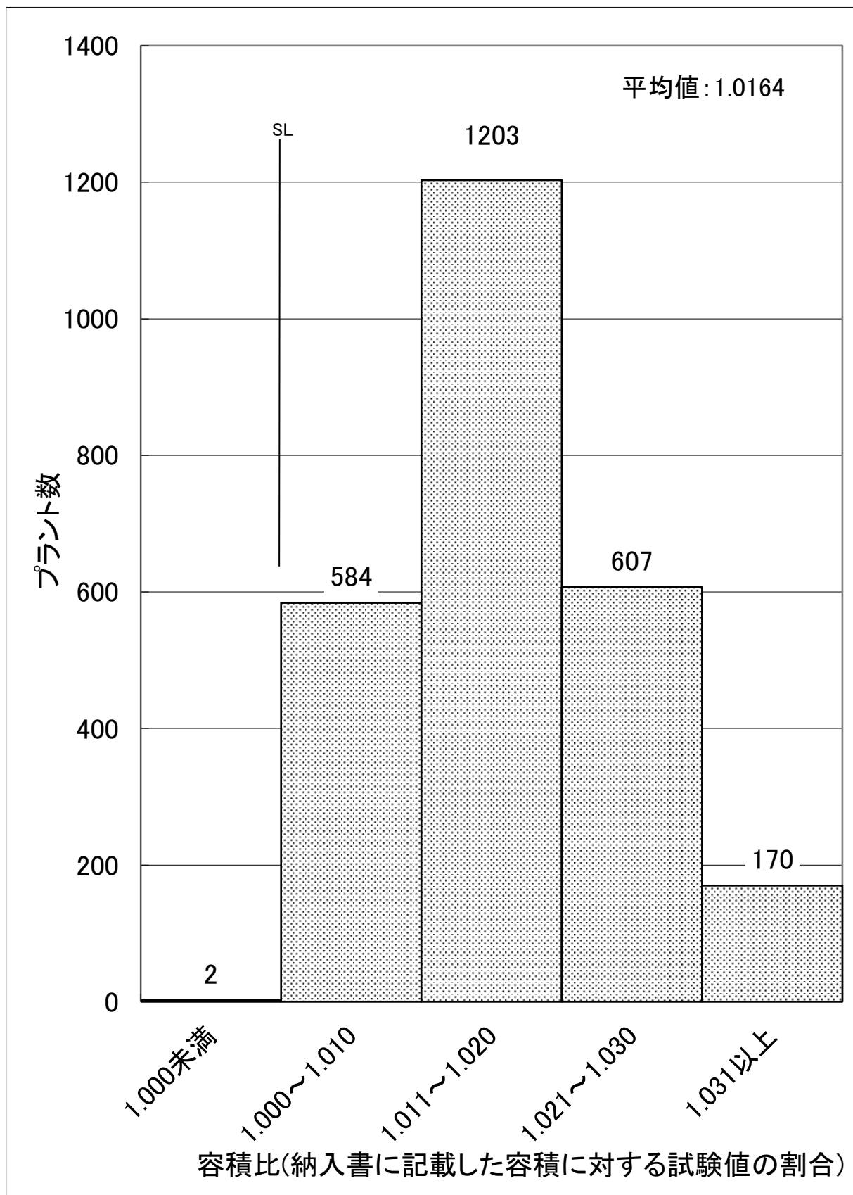
図-9 2019年度容積の適合性(実地調査) N=2,566
