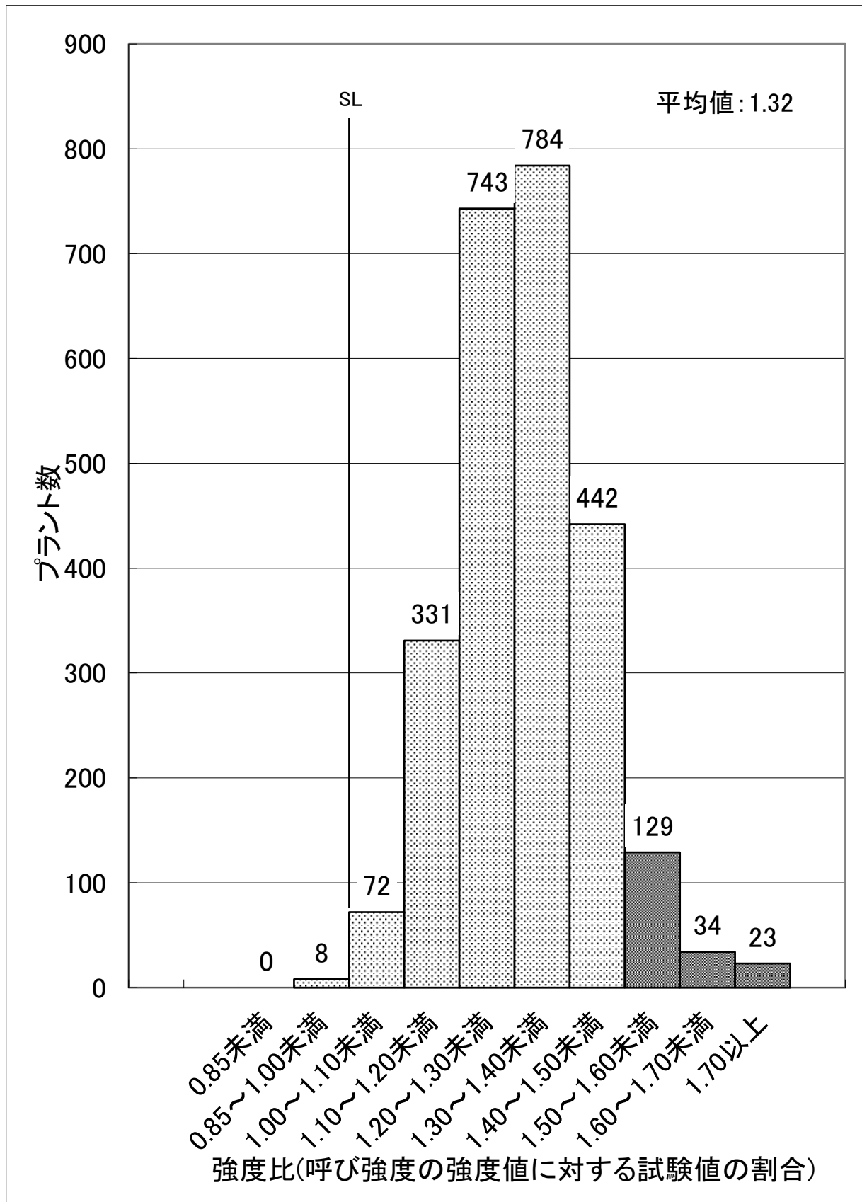
図-6 2019年度圧縮強度の適合性 N=2,566
